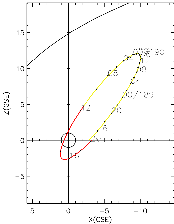
CLUSTER 2 orbit 2023 188 (07/07) 14:01 UT to 2023 190 (07/09) 20:11 UT
