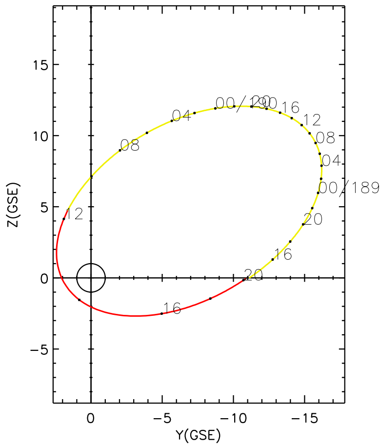
CLUSTER 2 orbit 2023 188 (07/07) 14:01 UT to 2023 190 (07/09) 20:11 UT
