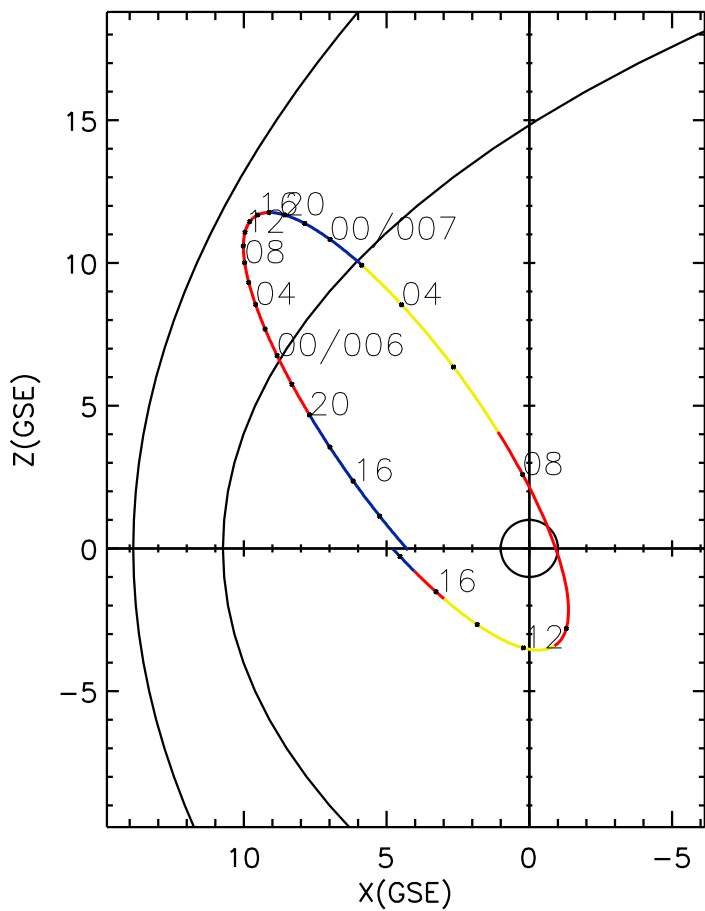
CLUSTER 2 orbit 2023 005 (01/05) 12:06 UT to 2023 007 (01/07) 18:26 UT
