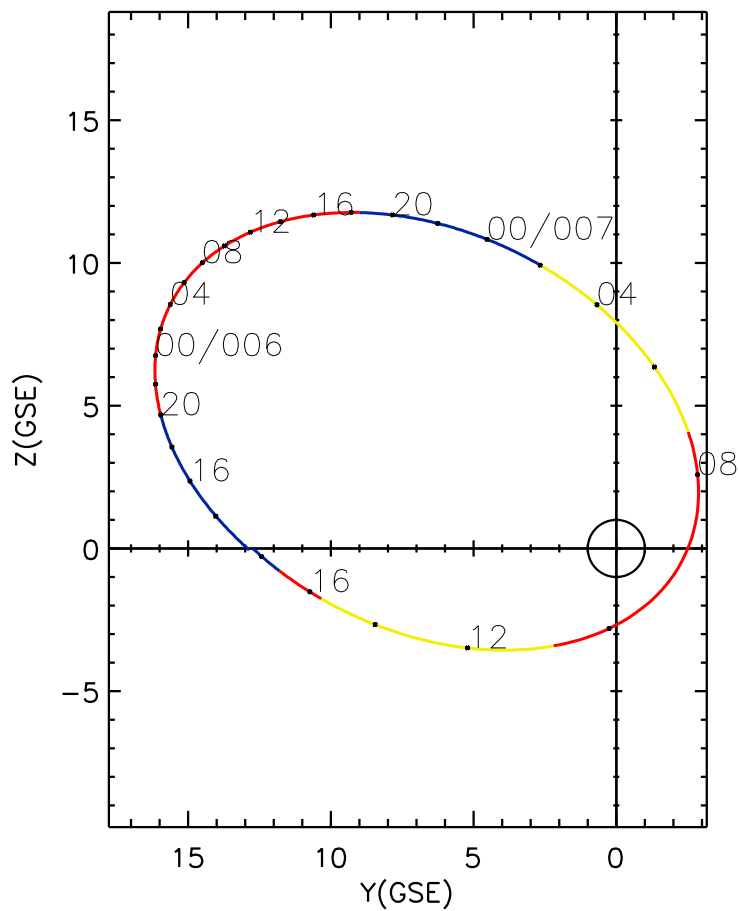
CLUSTER 2 orbit 2023 005 (01/05) 12:06 UT to 2023 007 (01/07) 18:26 UT
