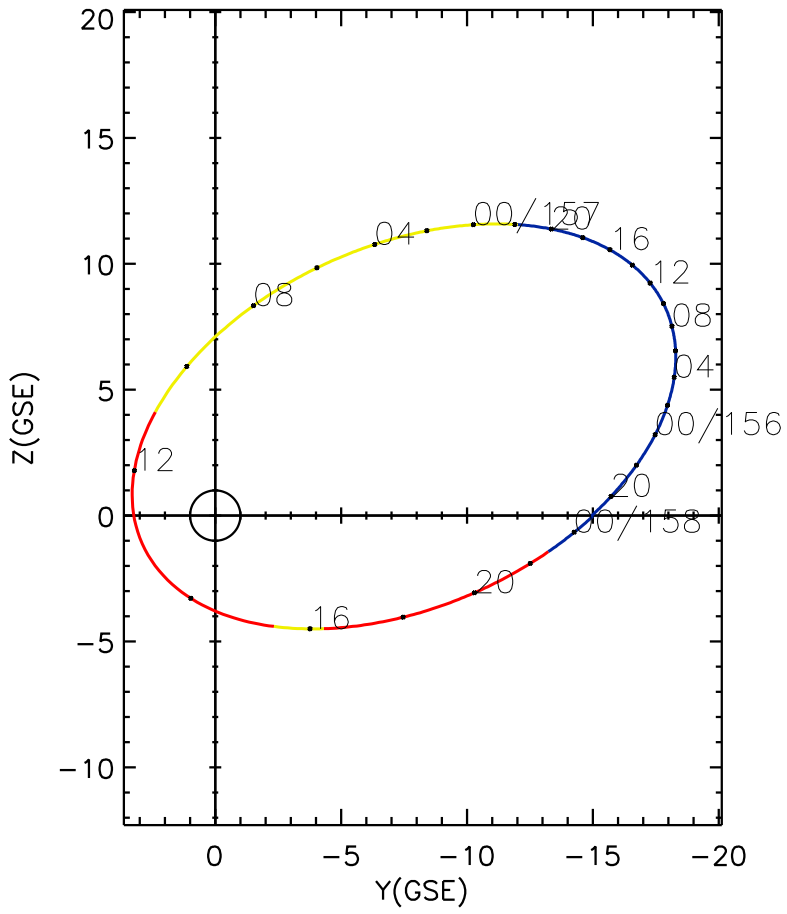
CLUSTER 2 orbit 2022 155 (06/04) 18:46 UT to 2022 158 (06/07) 01:01 UT
