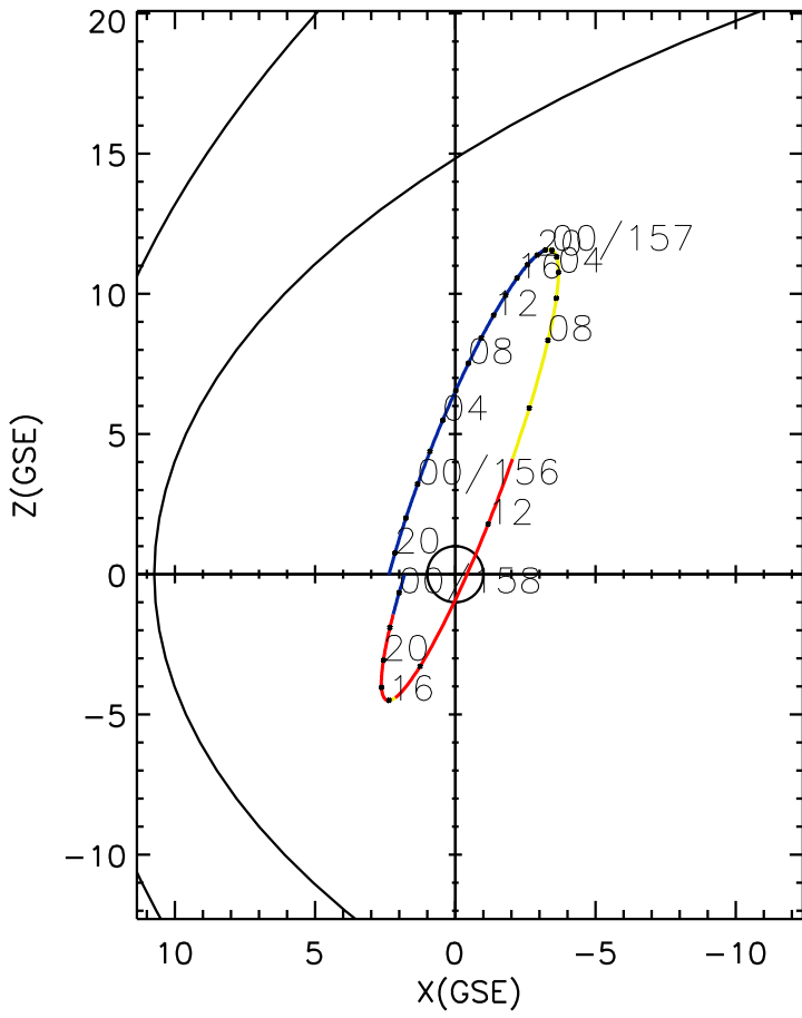
CLUSTER 2 orbit 2022 155 (06/04) 18:46 UT to 2022 158 (06/07) 01:01 UT
