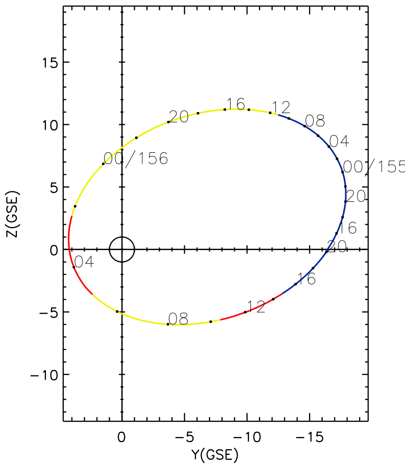
CLUSTER 2 orbit 2021 154 (06/03) 14:01 UT to 2021 156 (06/05) 20:16 UT
