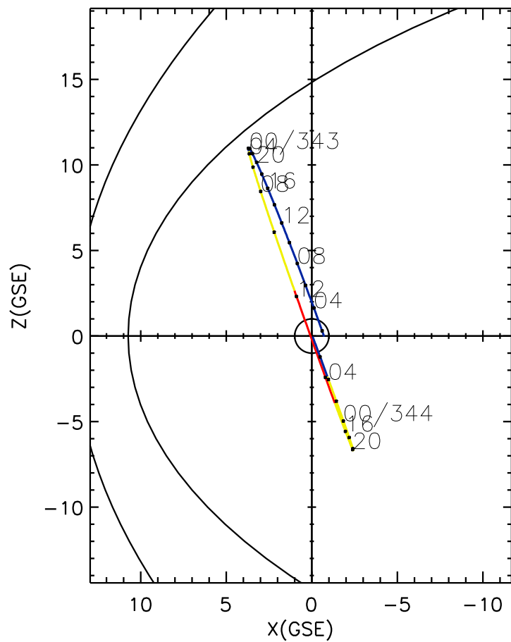
CLUSTER 2 orbit 2020 342 (12/07) 01:31 UT to 2020 344 (12/09) 07:46 UT
