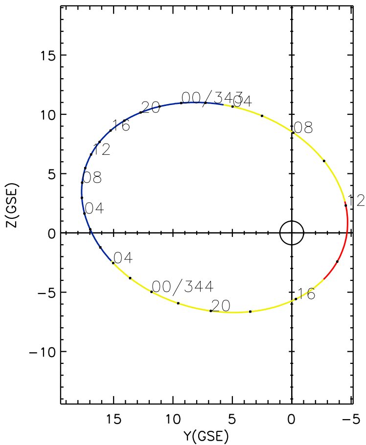
CLUSTER 2 orbit 2020 342 (12/07) 01:31 UT to 2020 344 (12/09) 07:46 UT
