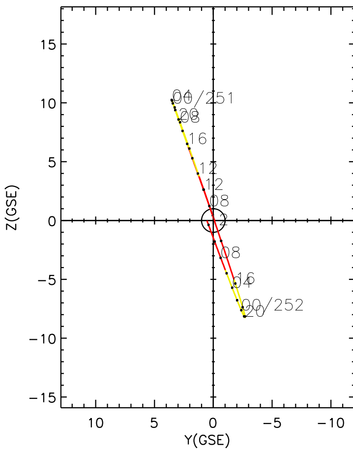
CLUSTER 2 orbit 2019 250 (09/07) 06:11 UT to 2019 252 (09/09) 12:31 UT
