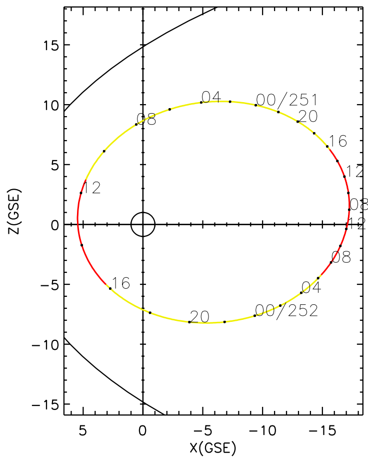
CLUSTER 2 orbit 2019 250 (09/07) 06:11 UT to 2019 252 (09/09) 12:31 UT
