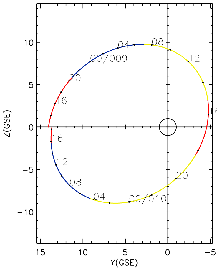
CLUSTER 2 orbit 2019 008 (01/08) 12:06 UT to 2019 010 (01/10) 18:16 UT
