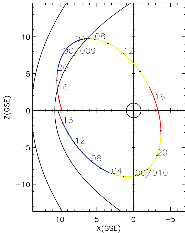
CLUSTER 2 orbit 2019 008 (01/08) 12:06 UT to 2019 010 (01/10) 18:16 UT
