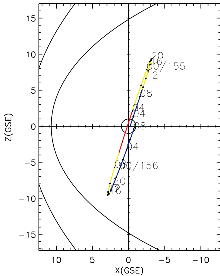
CLUSTER 2 orbit 2018 154 (06/03) 02:11 UT to 2018 156 (06/05) 08:31 UT
