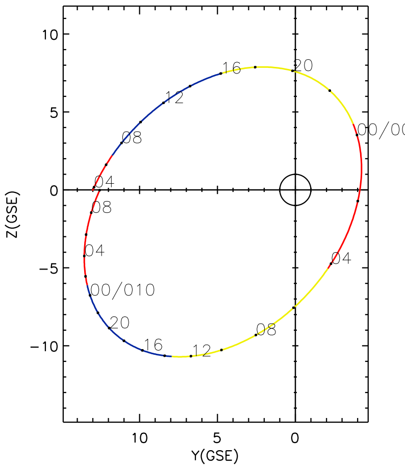
CLUSTER 2 orbit 2017 008 (01/08) 03:41 UT to 2017 010 (01/10) 10:01 UT
