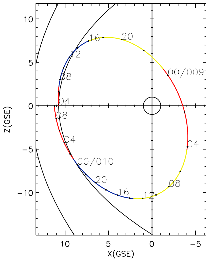
CLUSTER 2 orbit 2017 008 (01/08) 03:41 UT to 2017 010 (01/10) 10:01 UT
