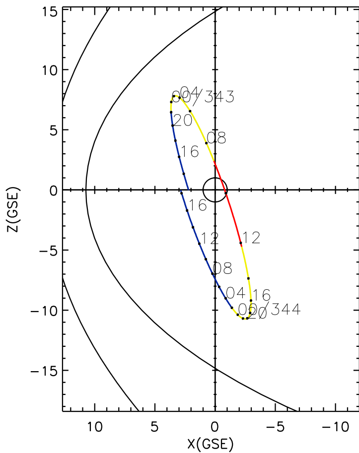
CLUSTER 2 orbit 2016 342 (12/07) 12:06 UT to 2016 344 (12/09) 18:21 UT
