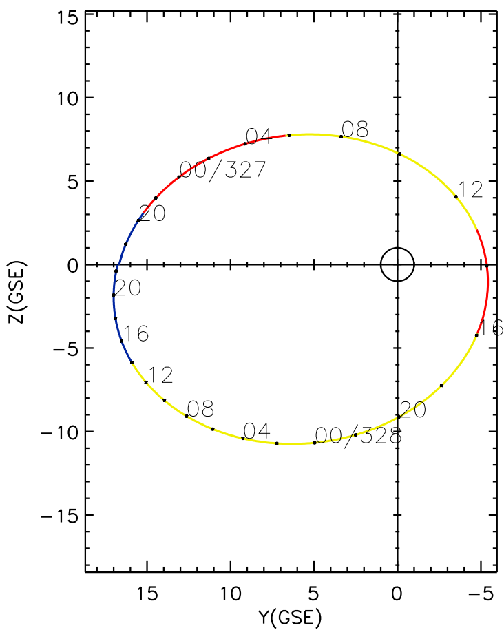
CLUSTER 2 orbit 2016 326 (11/21) 16:16 UT to 2016 328 (11/23) 22:31 UT
