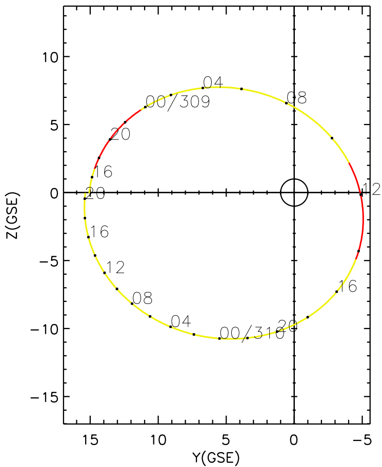
CLUSTER 2 orbit 2016 308 (11/03) 14:21 UT to 2016 310 (11/05) 20:36 UT
