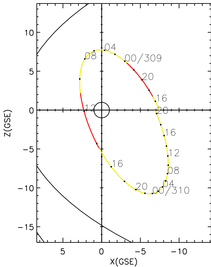
CLUSTER 2 orbit 2016 308 (11/03) 14:21 UT to 2016 310 (11/05) 20:36 UT
