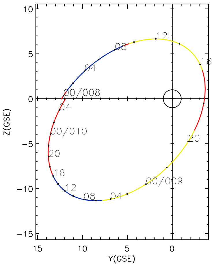
CLUSTER 2 orbit 2016 007 (01/07) 23:26 UT to 2016 010 (01/10) 05:46 UT
