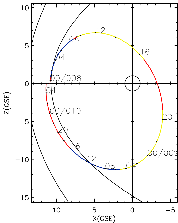
CLUSTER 2 orbit 2016 007 (01/07) 23:26 UT to 2016 010 (01/10) 05:46 UT
