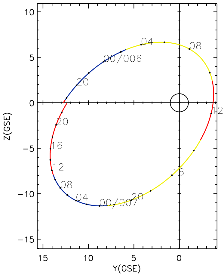
CLUSTER 2 orbit 2016 005 (01/05) 17:11 UT to 2016 007 (01/07) 23:26 UT
