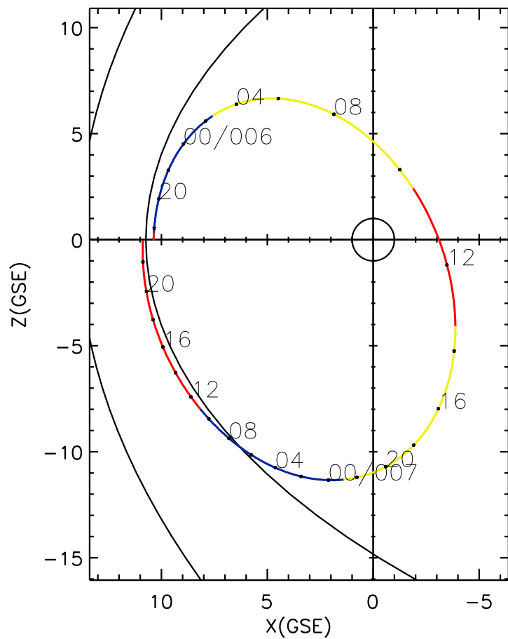
CLUSTER 2 orbit 2016 005 (01/05) 17:11 UT to 2016 007 (01/07) 23:26 UT
