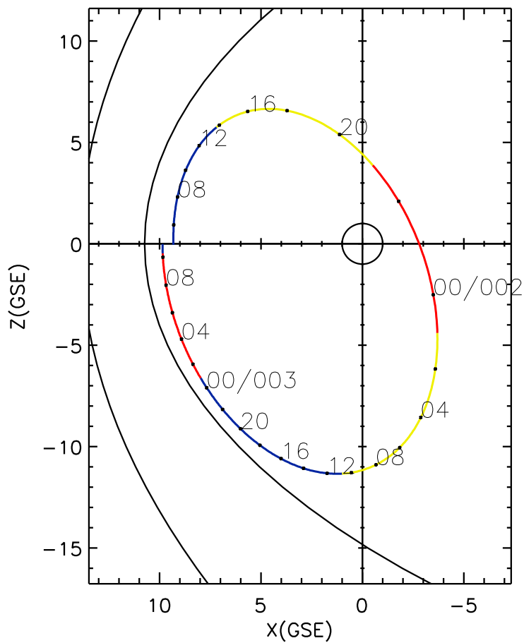
CLUSTER 2 orbit 2016 001 (01/01) 04:36 UT to 2016 003 (01/03) 10:56 UT
