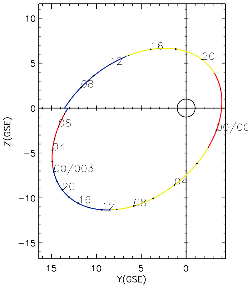
CLUSTER 2 orbit 2016 001 (01/01) 04:36 UT to 2016 003 (01/03) 10:56 UT
