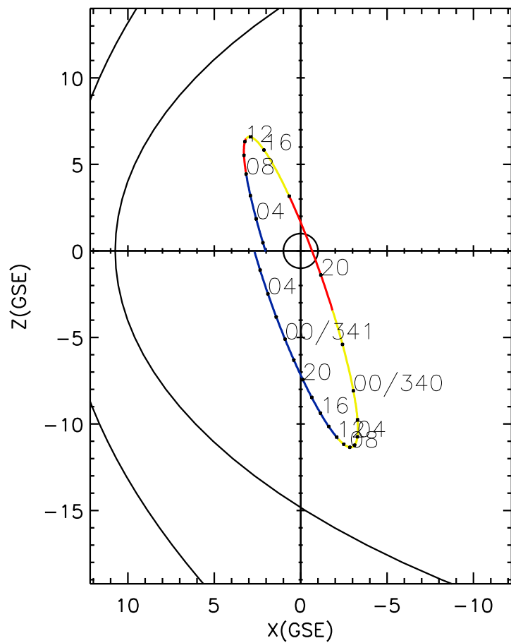
CLUSTER 2 orbit 2015 339 (12/05) 01:16 UT to 2015 341 (12/07) 07:31 UT
