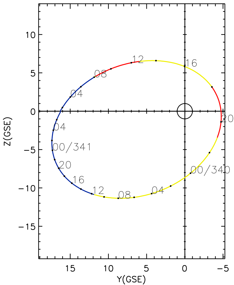
CLUSTER 2 orbit 2015 339 (12/05) 01:16 UT to 2015 341 (12/07) 07:31 UT
