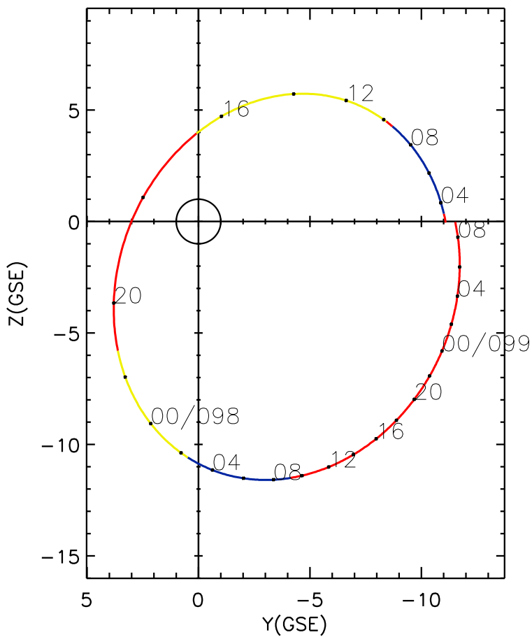
CLUSTER 2 orbit 2015 097 (04/07) 02:41 UT to 2015 099 (04/09) 09:01 UT
