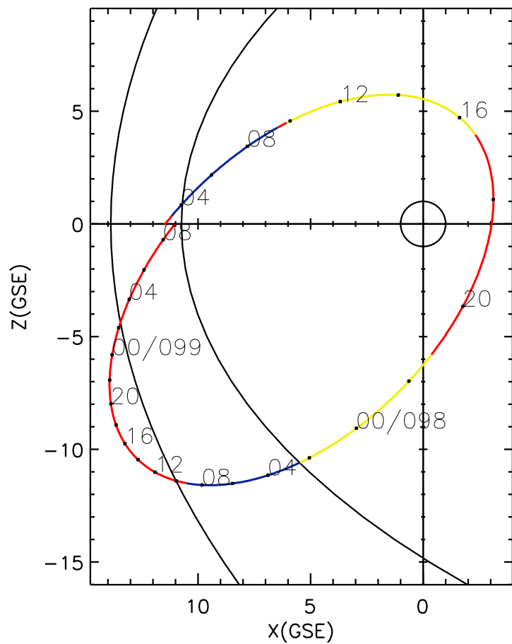
CLUSTER 2 orbit 2015 097 (04/07) 02:41 UT to 2015 099 (04/09) 09:01 UT
