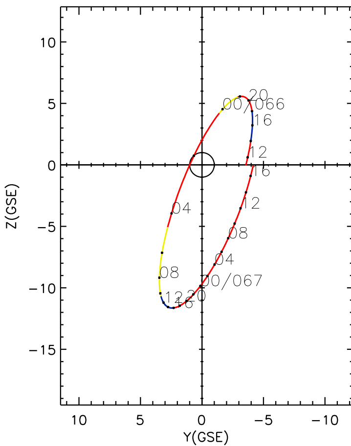
CLUSTER 2 orbit 2015 065 (03/06) 11:01 UT to 2015 067 (03/08) 17:16 UT
