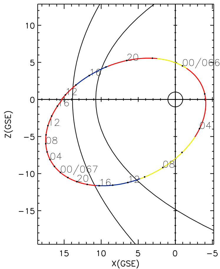
CLUSTER 2 orbit 2015 065 (03/06) 11:01 UT to 2015 067 (03/08) 17:16 UT
