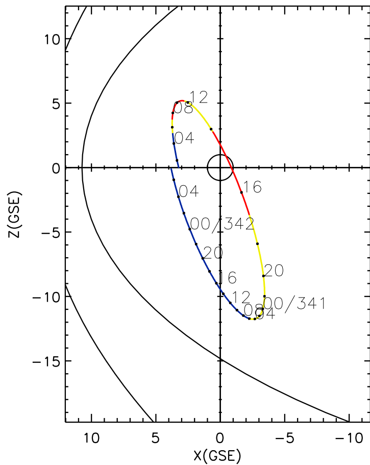
CLUSTER 2 orbit 2014 340 (12/06) 01:06 UT to 2014 342 (12/08) 07:21 UT
