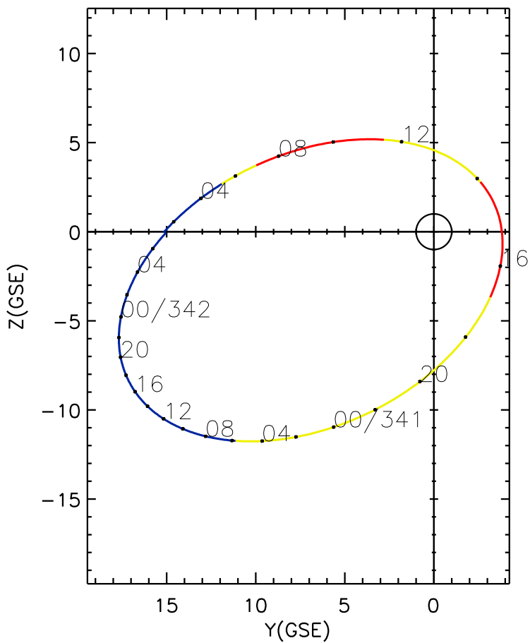
CLUSTER 2 orbit 2014 340 (12/06) 01:06 UT to 2014 342 (12/08) 07:21 UT
