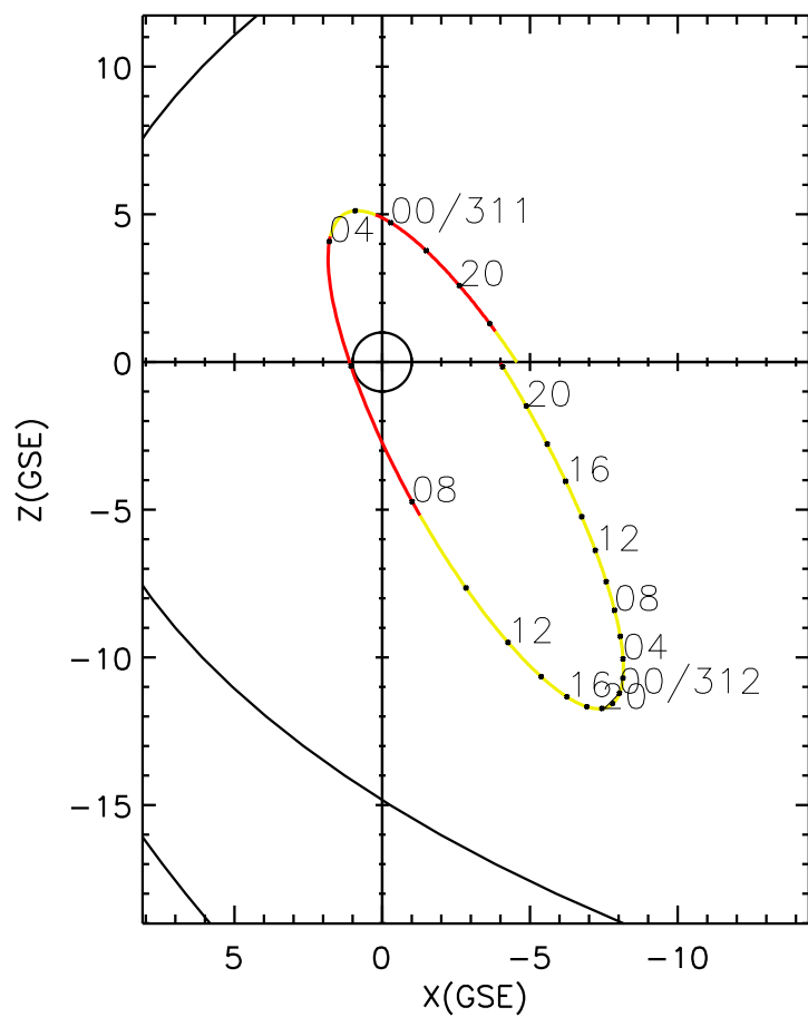
CLUSTER 2 orbit 2014 310 (11/06) 16:01 UT to 2014 312 (11/08) 22:11 UT
