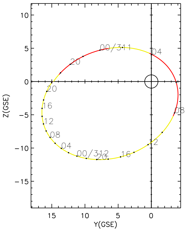
CLUSTER 2 orbit 2014 310 (11/06) 16:01 UT to 2014 312 (11/08) 22:11 UT
