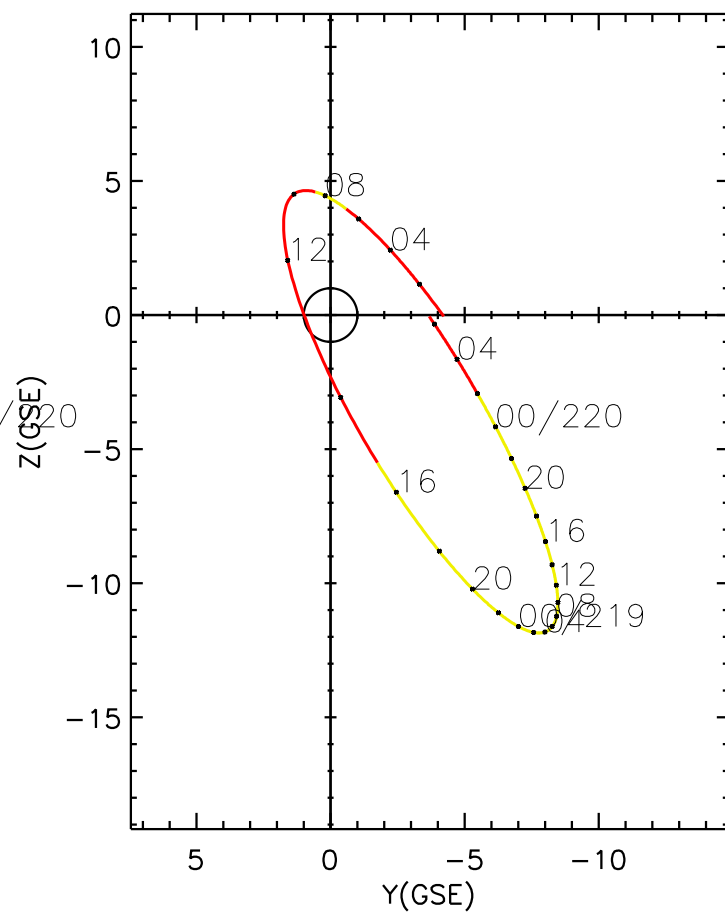
CLUSTER 2 orbit 2014 218 (08/06) 00:11 UT to 2014 220 (08/08) 06:26 UT
