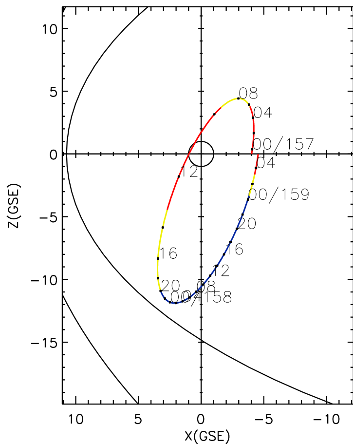
CLUSTER 2 orbit 2014 156 (06/05) 23:26 UT to 2014 159 (06/08) 05:41 UT
