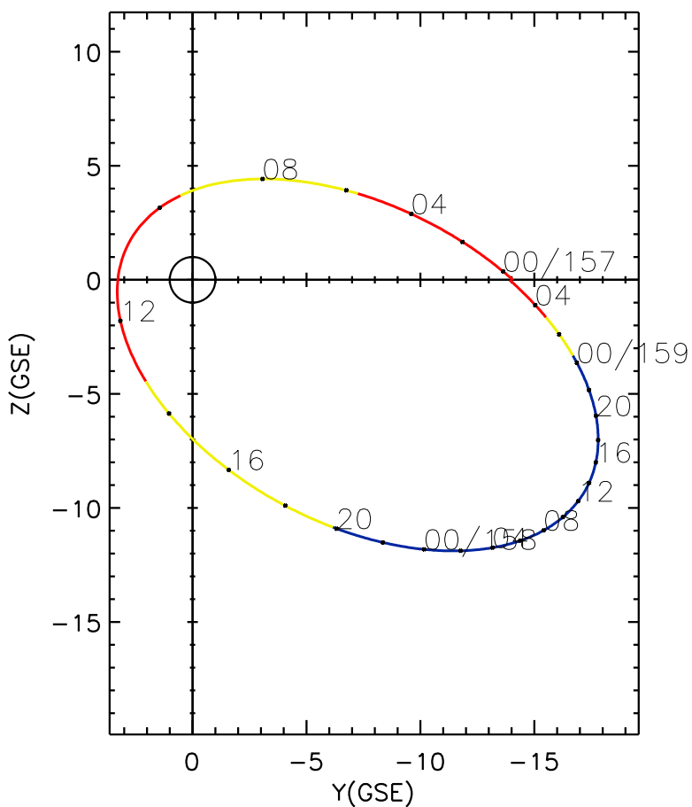
CLUSTER 2 orbit 2014 156 (06/05) 23:26 UT to 2014 159 (06/08) 05:41 UT
