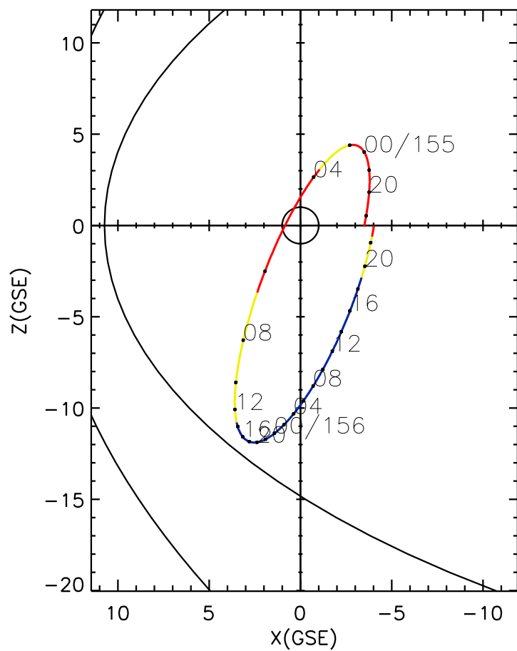
CLUSTER 2 orbit 2014 154 (06/03) 17:06 UT to 2014 156 (06/05) 23:26 UT
