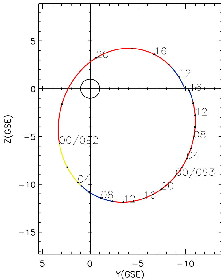
CLUSTER 2 orbit 2014 091 (04/01) 10:01 UT to 2014 093 (04/03) 16:16 UT
