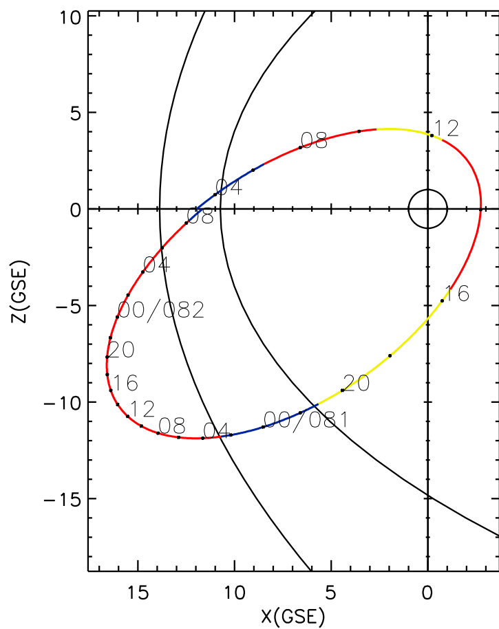
CLUSTER 2 orbit 2014 080 (03/21) 02:51 UT to 2014 082 (03/23) 09:06 UT
