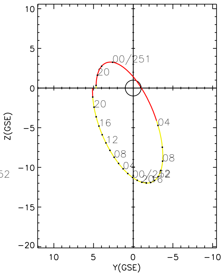
CLUSTER 2 orbit 2013 250 (09/07) 17:26 UT to 2013 252 (09/09) 23:41 UT
