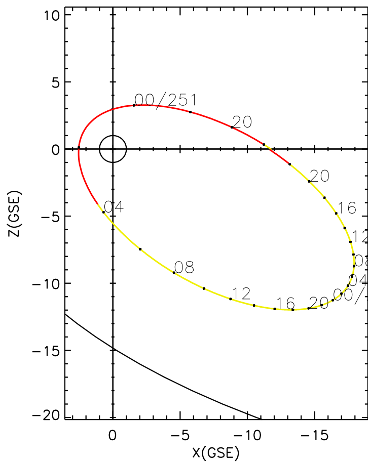
CLUSTER 2 orbit 2013 250 (09/07) 17:26 UT to 2013 252 (09/09) 23:41 UT
