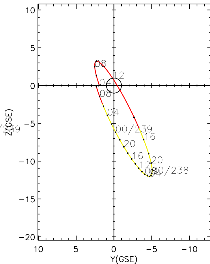
CLUSTER 2 orbit 2013 237 (08/25) 03:56 UT to 2013 239 (08/27) 10:11 UT
