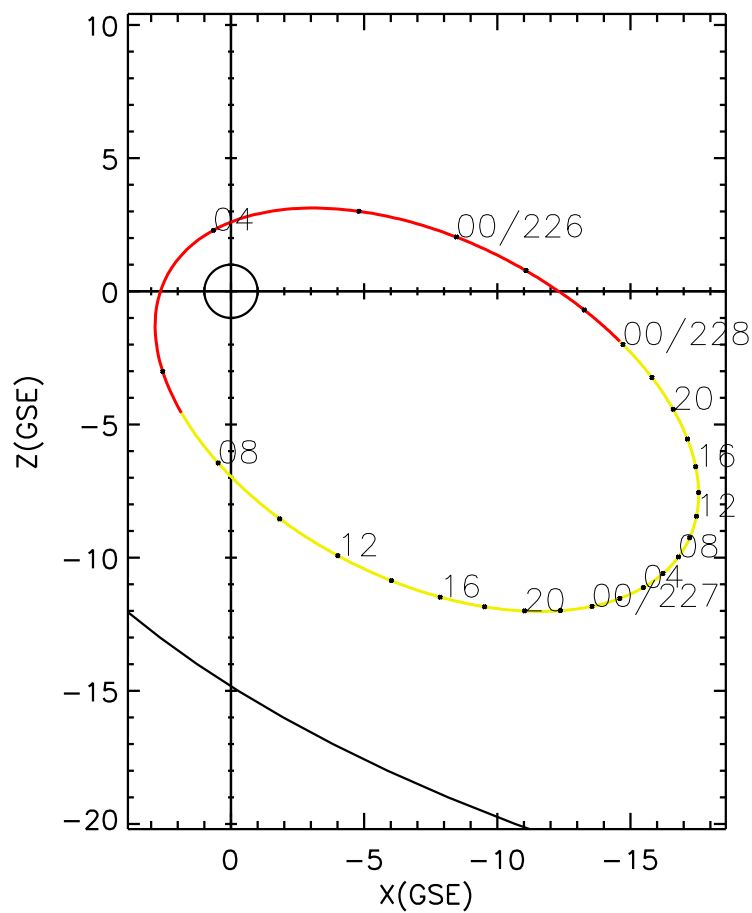
CLUSTER 2 orbit 2013 225 (08/13) 20:46 UT to 2013 228 (08/16) 03:01 UT
