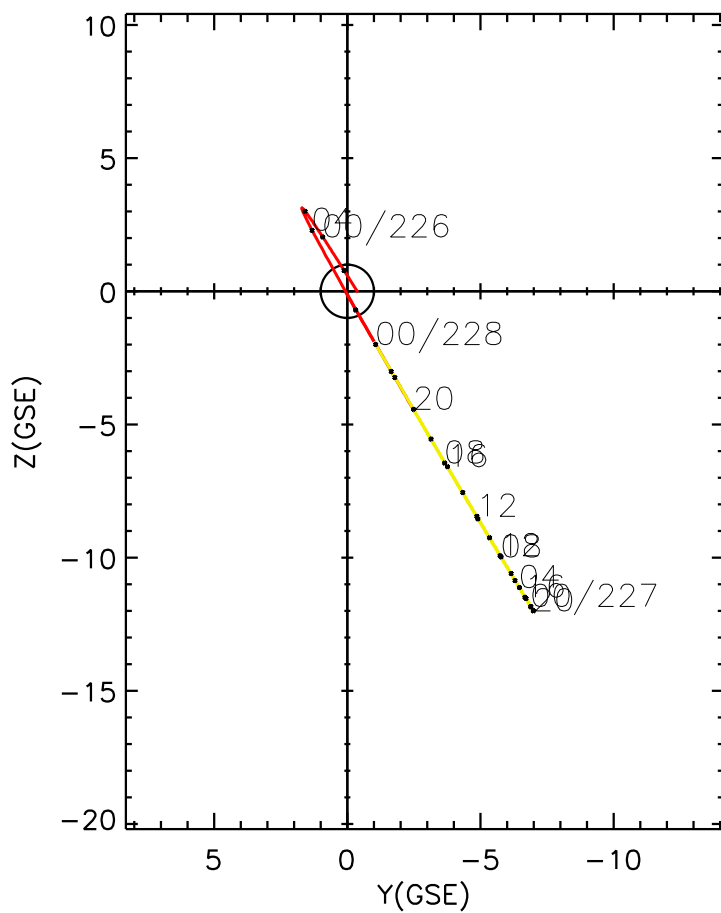
CLUSTER 2 orbit 2013 225 (08/13) 20:46 UT to 2013 228 (08/16) 03:01 UT
