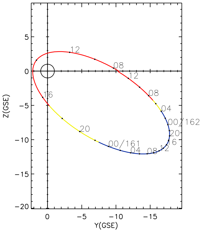
CLUSTER 2 orbit 2013 160 (06/09) 07:16 UT to 2013 162 (06/11) 13:31 UT
