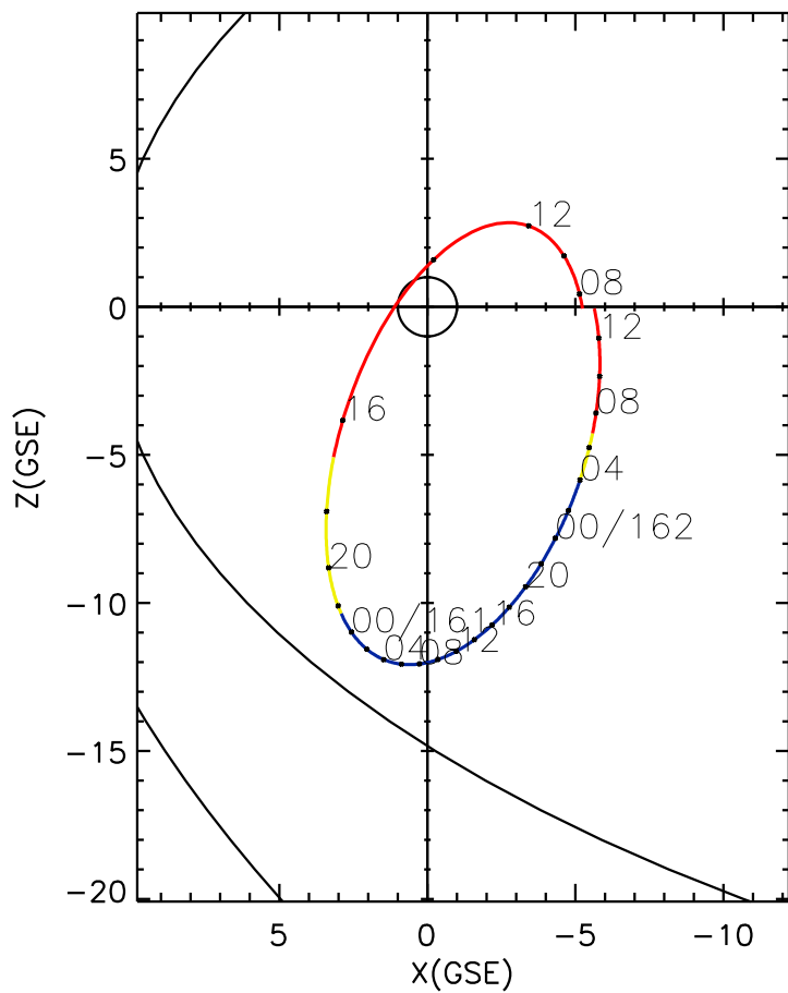
CLUSTER 2 orbit 2013 160 (06/09) 07:16 UT to 2013 162 (06/11) 13:31 UT
