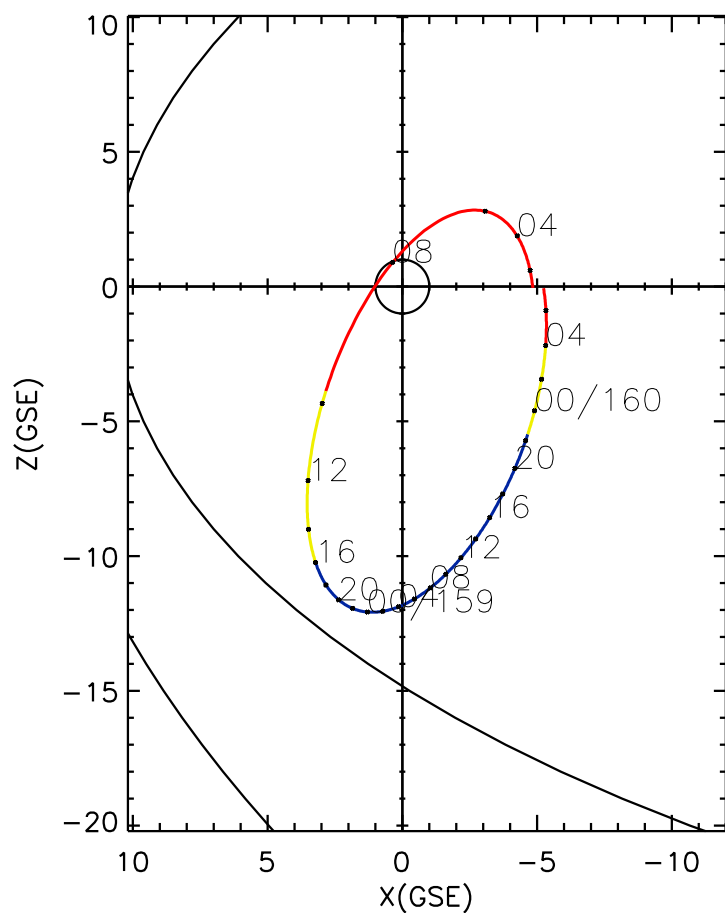
CLUSTER 2 orbit 2013 158 (06/07) 01:01 UT to 2013 160 (06/09) 07:16 UT
