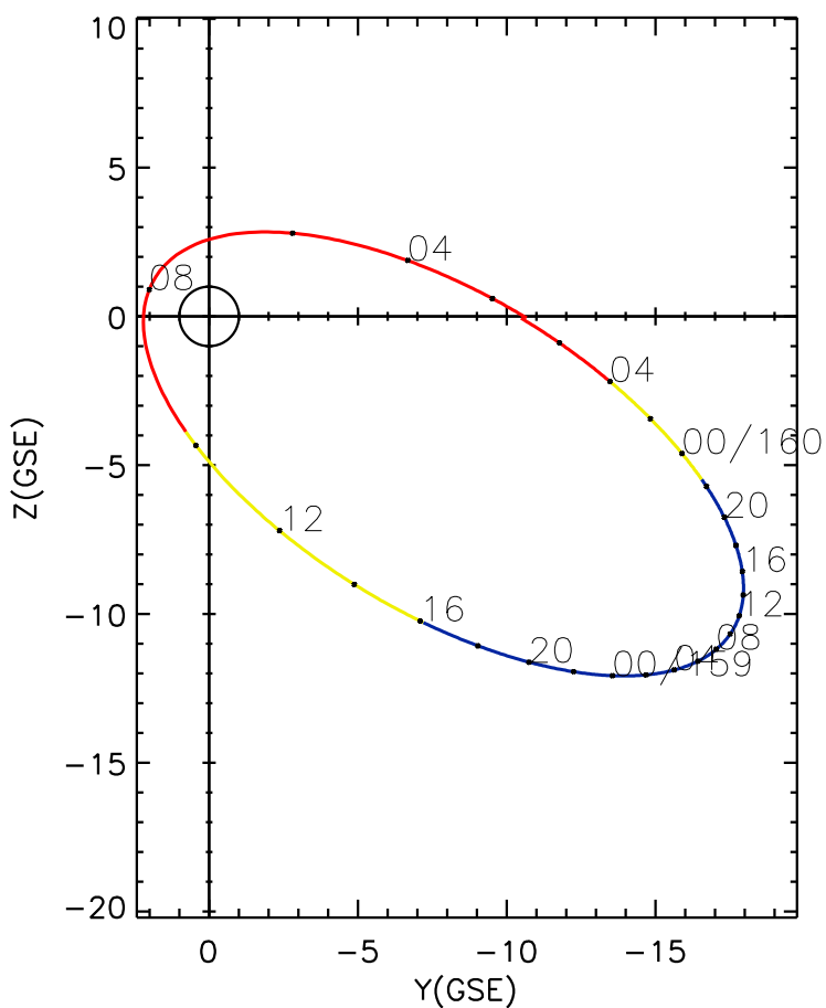
CLUSTER 2 orbit 2013 158 (06/07) 01:01 UT to 2013 160 (06/09) 07:16 UT
