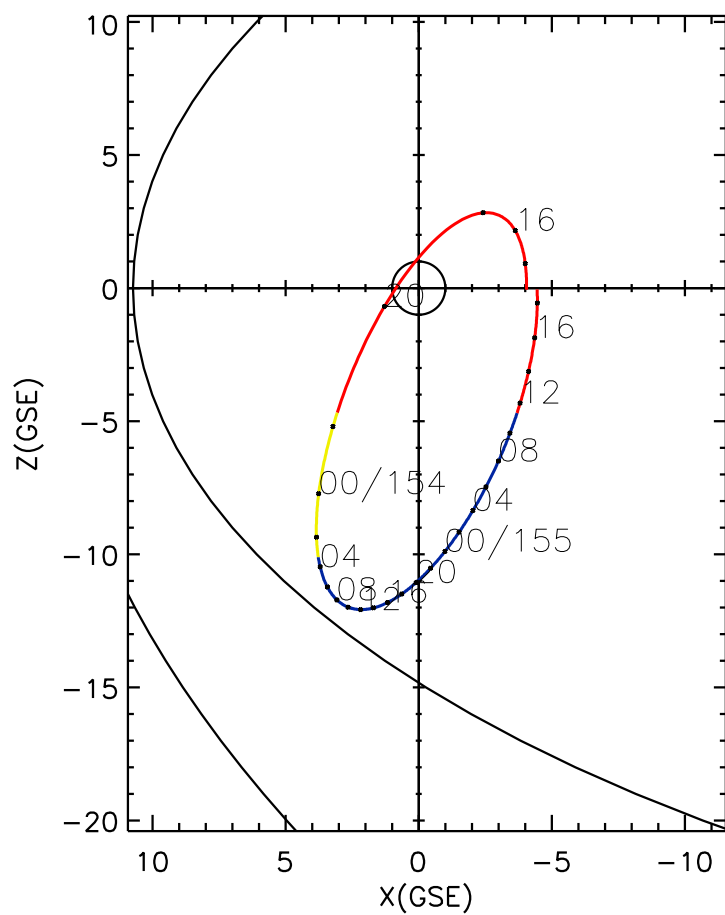
CLUSTER 2 orbit 2013 153 (06/02) 12:31 UT to 2013 155 (06/04) 18:46 UT
