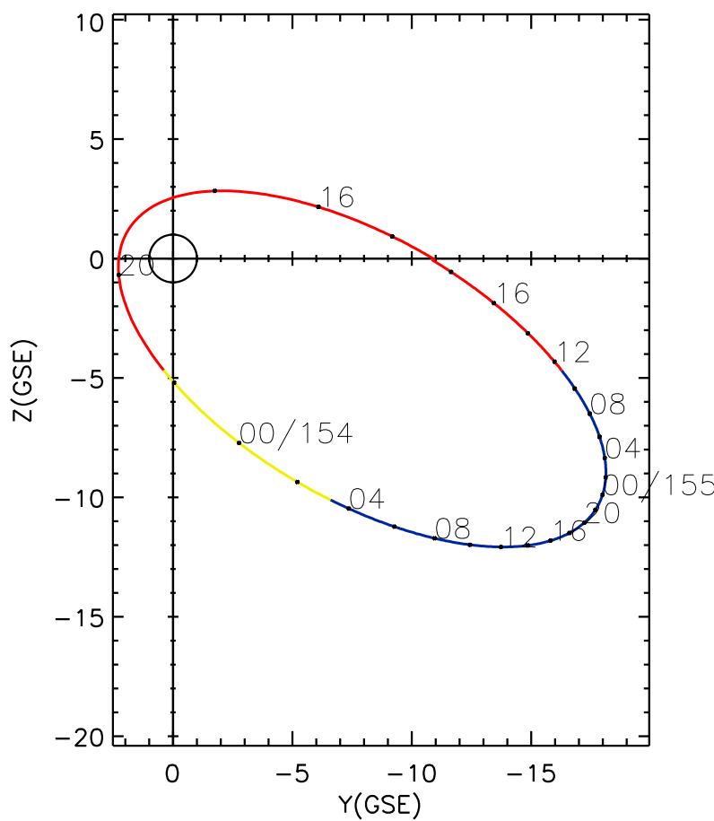
CLUSTER 2 orbit 2013 153 (06/02) 12:31 UT to 2013 155 (06/04) 18:46 UT
