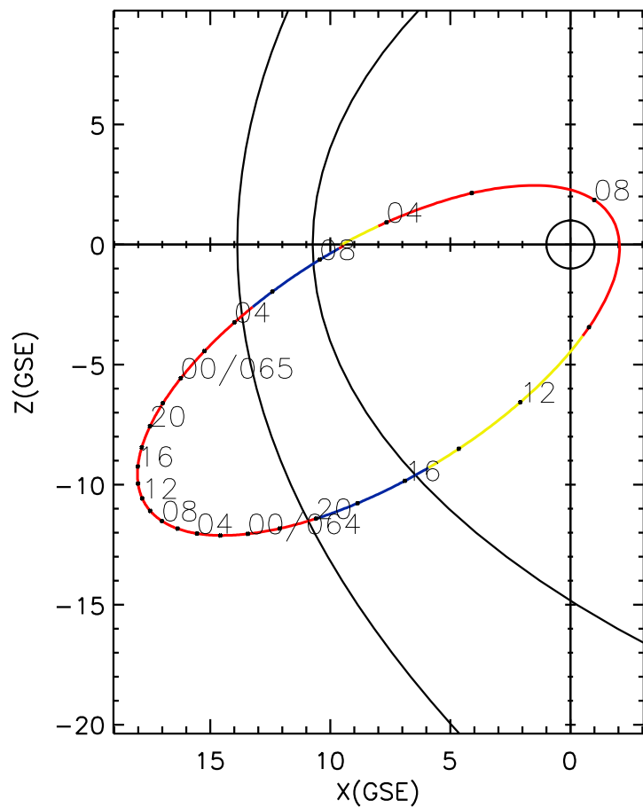
CLUSTER 2 orbit 2013 063 (03/04) 02:36 UT to 2013 065 (03/06) 08:51 UT
