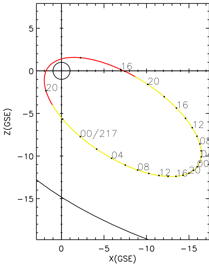
CLUSTER 2 orbit 2012 216 (08/03) 15:46 UT to 2012 218 (08/05) 22:01 UT
