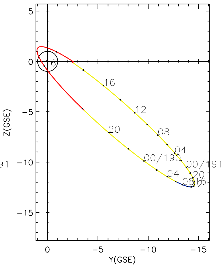
CLUSTER 2 orbit 2012 189 (07/07) 12:46 UT to 2012 191 (07/09) 19:01 UT
