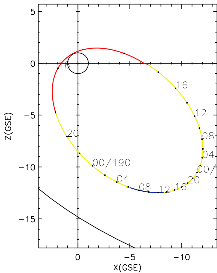
CLUSTER 2 orbit 2012 189 (07/07) 12:46 UT to 2012 191 (07/09) 19:01 UT
