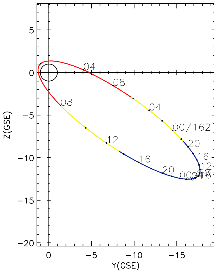
CLUSTER 2 orbit 2012 160 (06/08) 03:36 UT to 2012 162 (06/10) 09:51 UT
