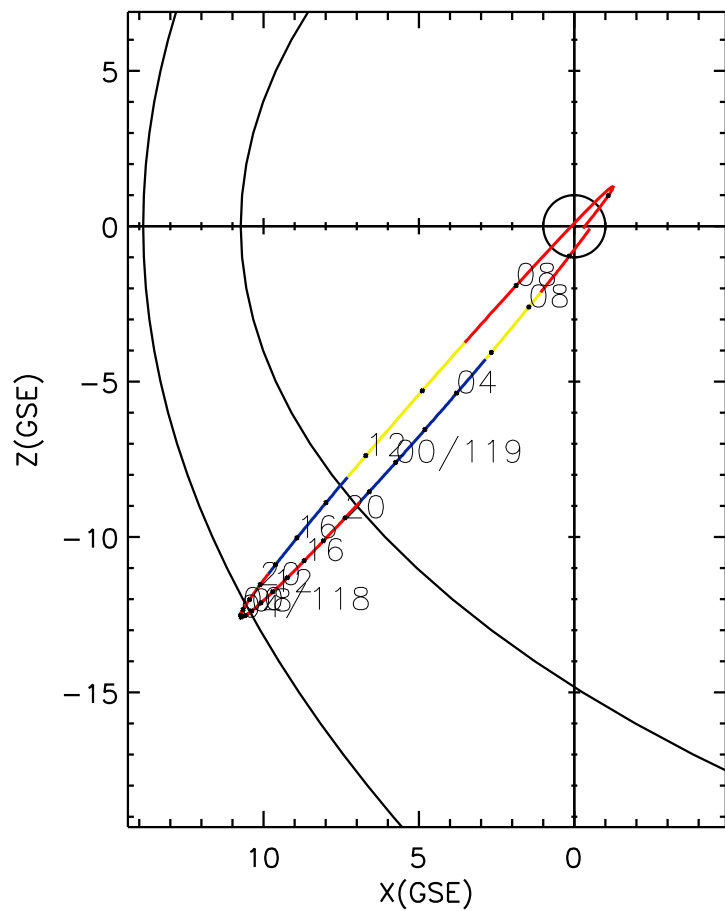
CLUSTER 2 orbit 2012 117 (04/26) 04:46 UT to 2012 119 (04/28) 11:01 UT
