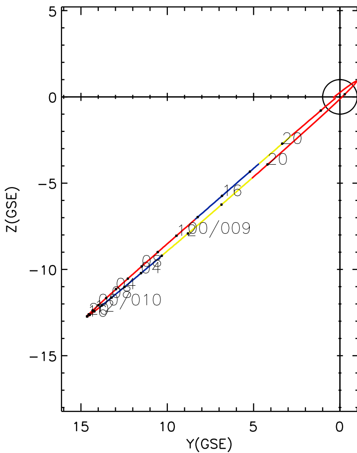
CLUSTER 2 orbit 2012 008 (01/08) 16:26 UT to 2012 010 (01/10) 22:41 UT
