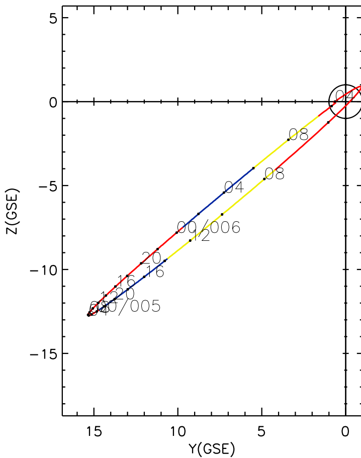
CLUSTER 2 orbit 2012 004 (01/04) 03:56 UT to 2012 006 (01/06) 10:11 UT
