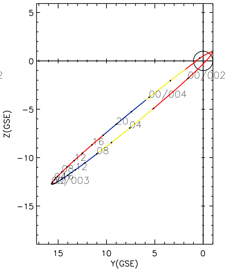
CLUSTER 2 orbit 2012 001 (01/01) 21:41 UT to 2012 004 (01/04) 03:56 UT
