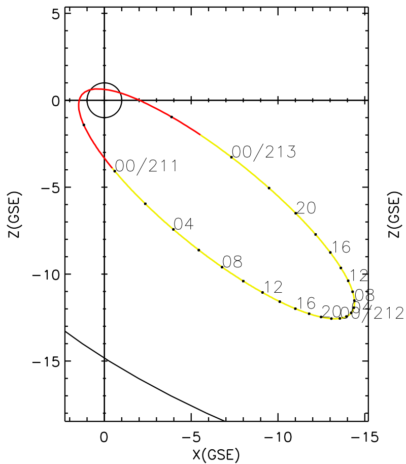
CLUSTER 2 orbit 2011 210 (07/29) 20:11 UT to 2011 213 (08/01) 02:36 UT
