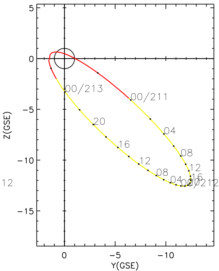
CLUSTER 2 orbit 2011 210 (07/29) 20:11 UT to 2011 213 (08/01) 02:36 UT
