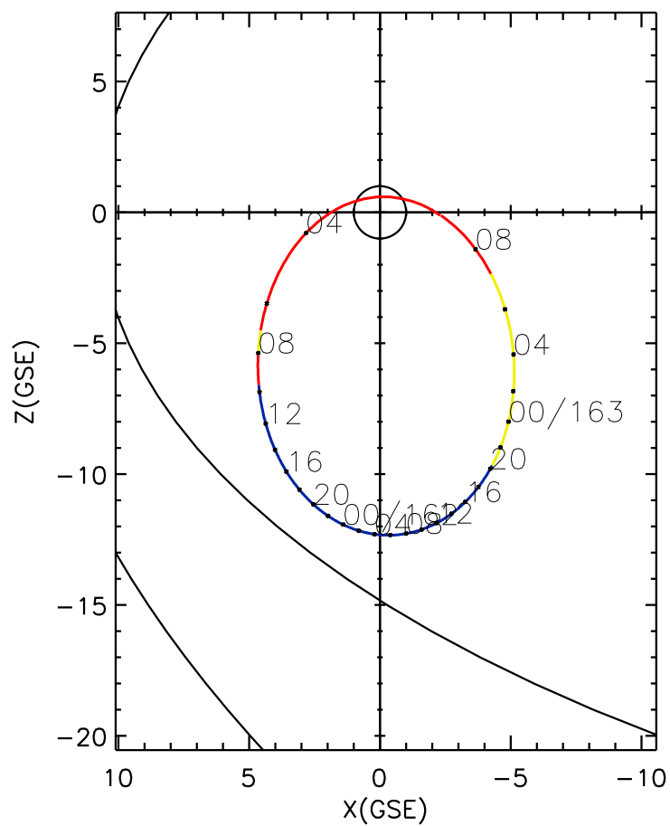
CLUSTER 2 orbit 2011 161 (06/10) 02:36 UT to 2011 163 (06/12) 08:51 UT
