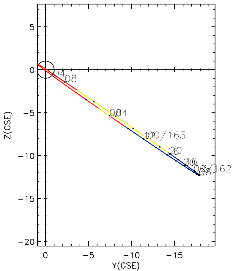
CLUSTER 2 orbit 2011 161 (06/10) 02:36 UT to 2011 163 (06/12) 08:51 UT
