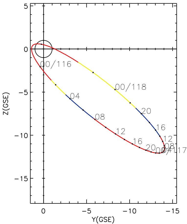
CLUSTER 2 orbit 2011 115 (04/25) 21:36 UT to 2011 118 (04/28) 03:51 UT
