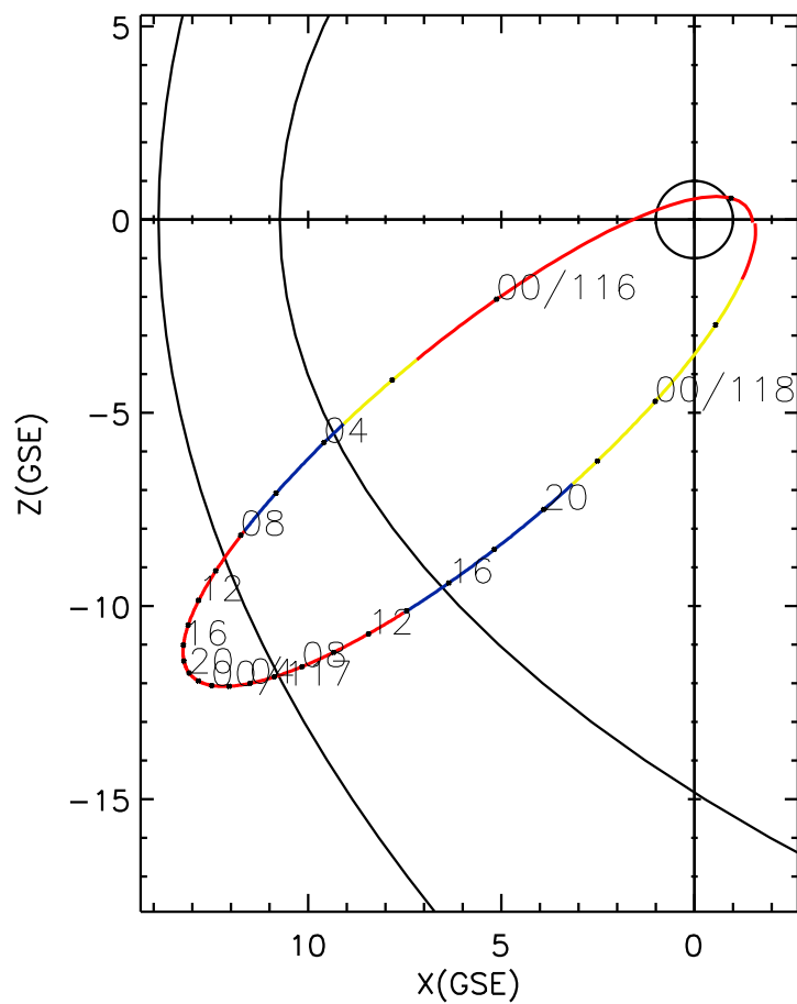
CLUSTER 2 orbit 2011 115 (04/25) 21:36 UT to 2011 118 (04/28) 03:51 UT
