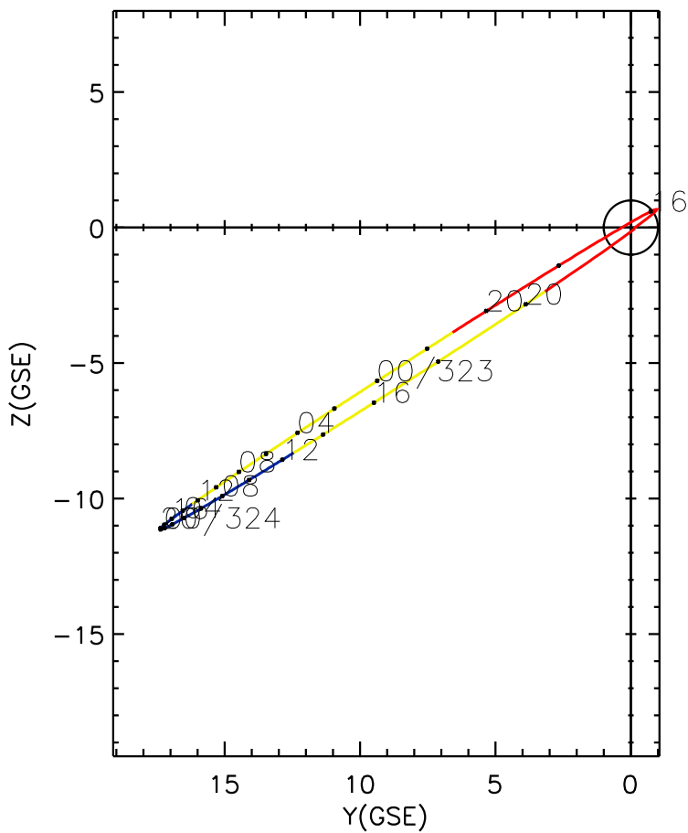
CLUSTER 2 orbit 2010 322 (11/18) 15:21 UT to 2010 324 (11/20) 21:36 UT
