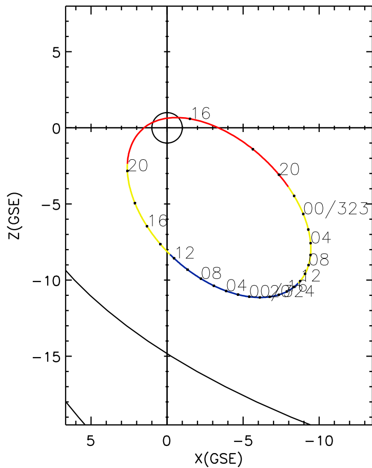
CLUSTER 2 orbit 2010 322 (11/18) 15:21 UT to 2010 324 (11/20) 21:36 UT
