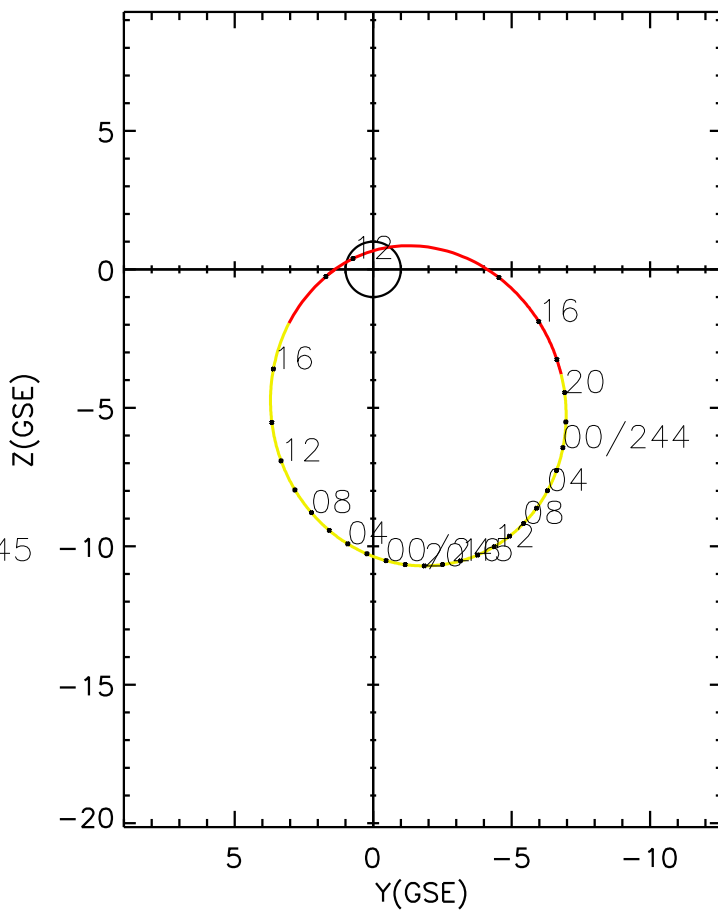
CLUSTER 2 orbit 2010 243 (08/31) 11:46 UT to 2010 245 (09/02) 18:06 UT
