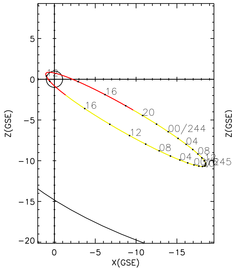
CLUSTER 2 orbit 2010 243 (08/31) 11:46 UT to 2010 245 (09/02) 18:06 UT
