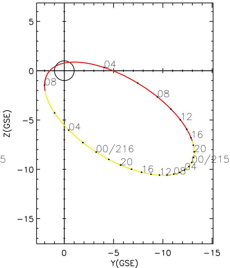
CLUSTER 2 orbit 2010 214 (08/02) 02:26 UT to 2010 216 (08/04) 08:36 UT
