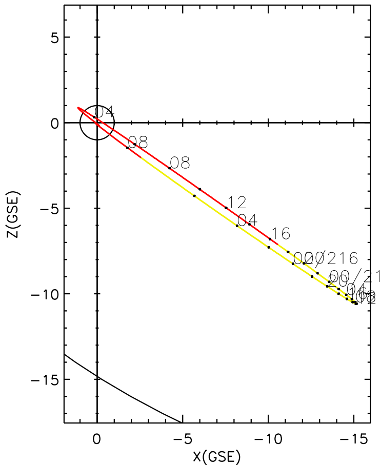
CLUSTER 2 orbit 2010 214 (08/02) 02:26 UT to 2010 216 (08/04) 08:36 UT
