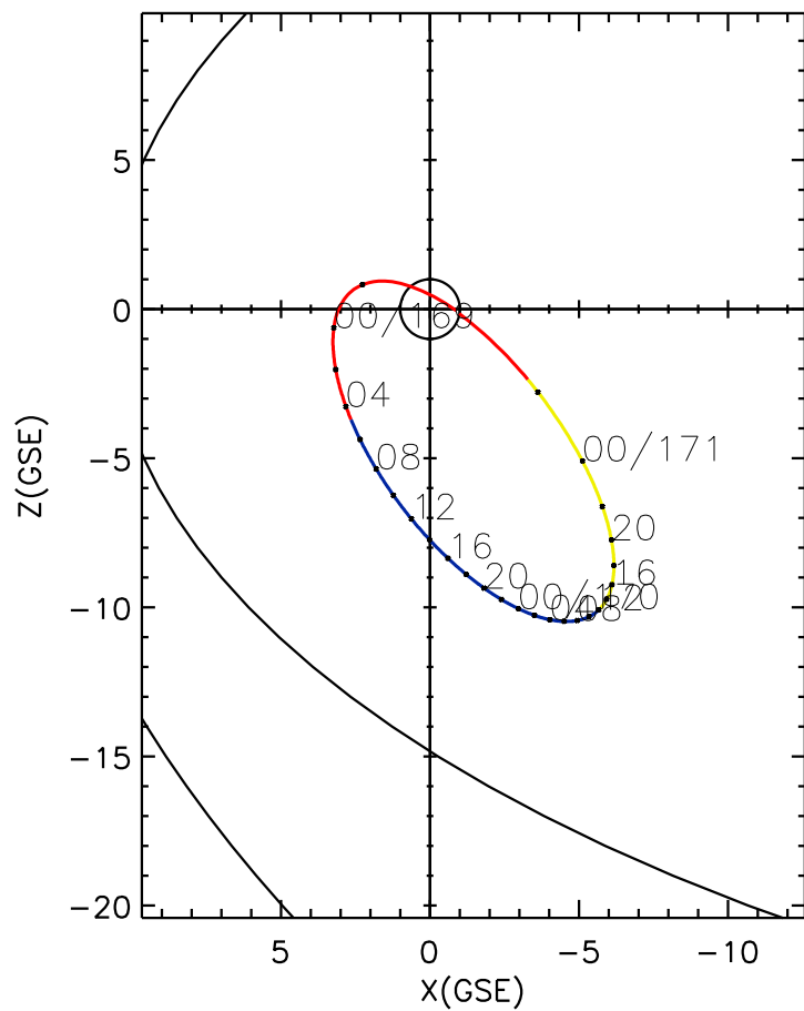
CLUSTER 2 orbit 2010 168 (06/17) 21:01 UT to 2010 171 (06/20) 03:16 UT
