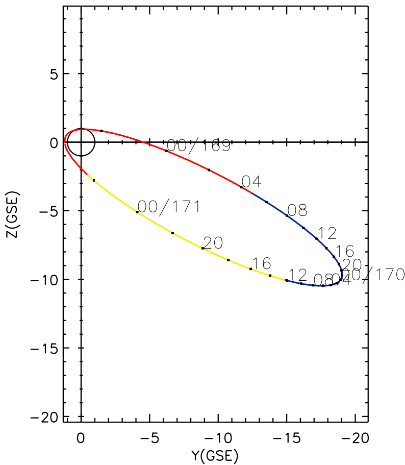
CLUSTER 2 orbit 2010 168 (06/17) 21:01 UT to 2010 171 (06/20) 03:16 UT
