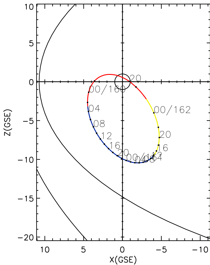
CLUSTER 2 orbit 2010 159 (06/08) 19:56 UT to 2010 162 (06/11) 02:11 UT
