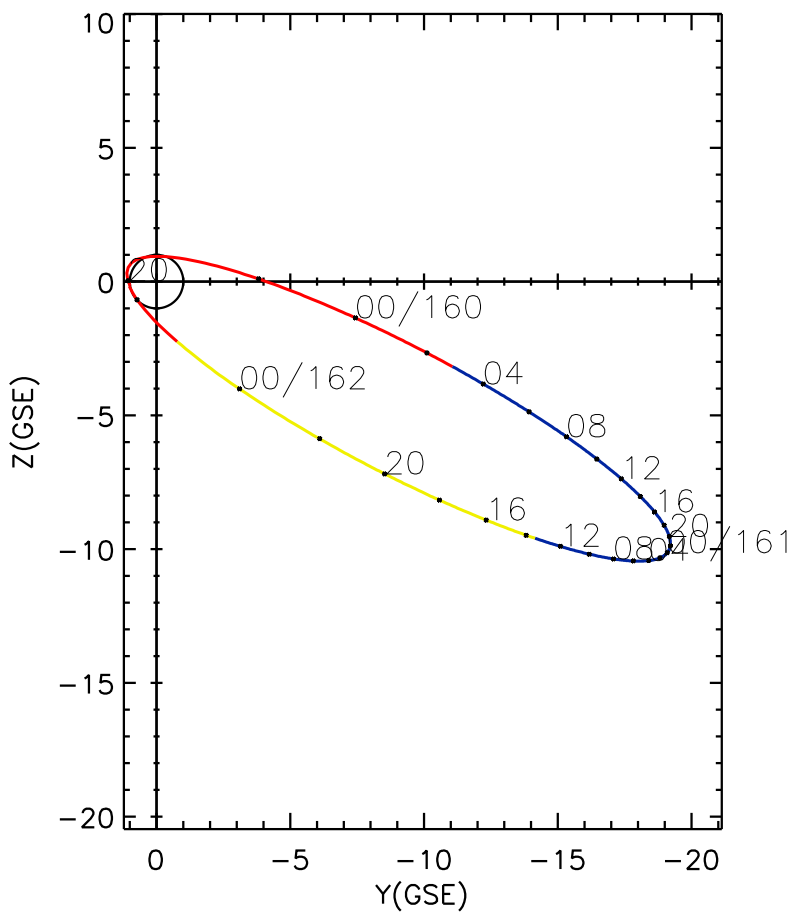
CLUSTER 2 orbit 2010 159 (06/08) 19:56 UT to 2010 162 (06/11) 02:11 UT
