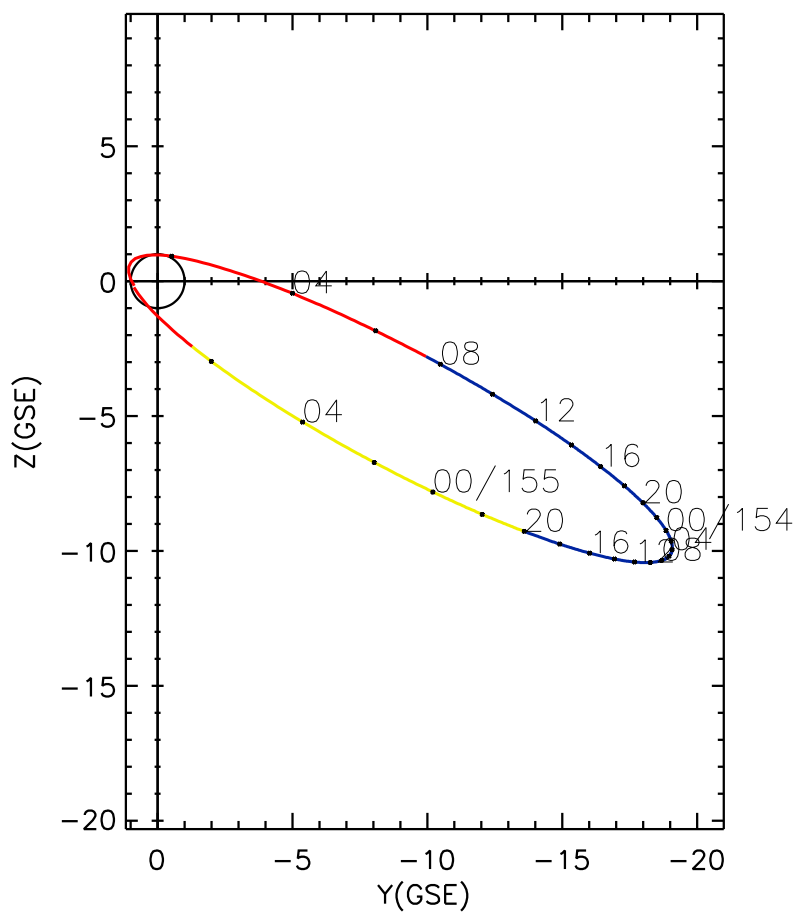
CLUSTER 2 orbit 2010 153 (06/02) 01:06 UT to 2010 155 (06/04) 07:21 UT
