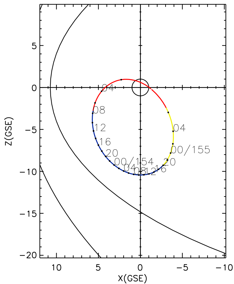
CLUSTER 2 orbit 2010 153 (06/02) 01:06 UT to 2010 155 (06/04) 07:21 UT
