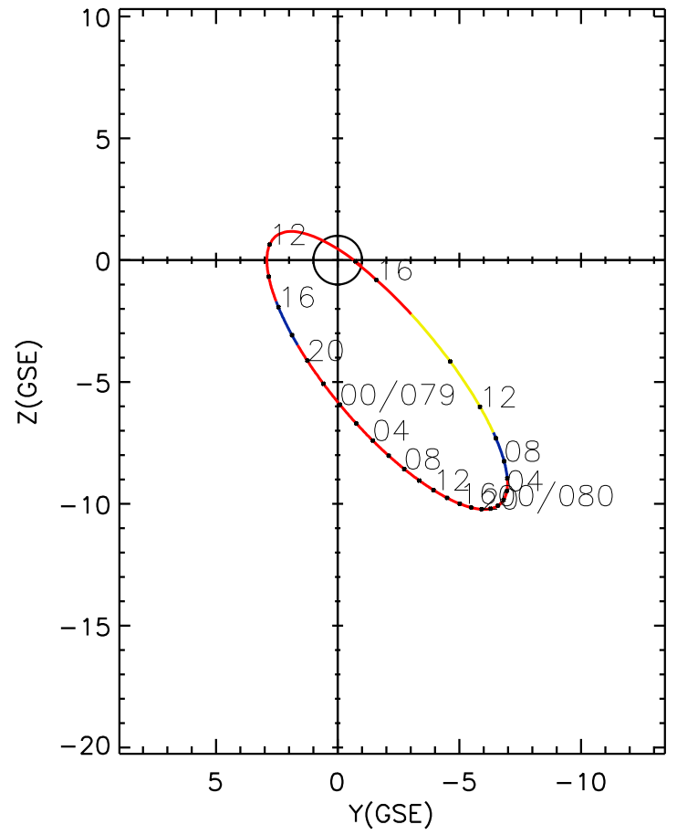
CLUSTER 2 orbit 2010 078 (03/19) 09:56 UT to 2010 080 (03/21) 16:16 UT
