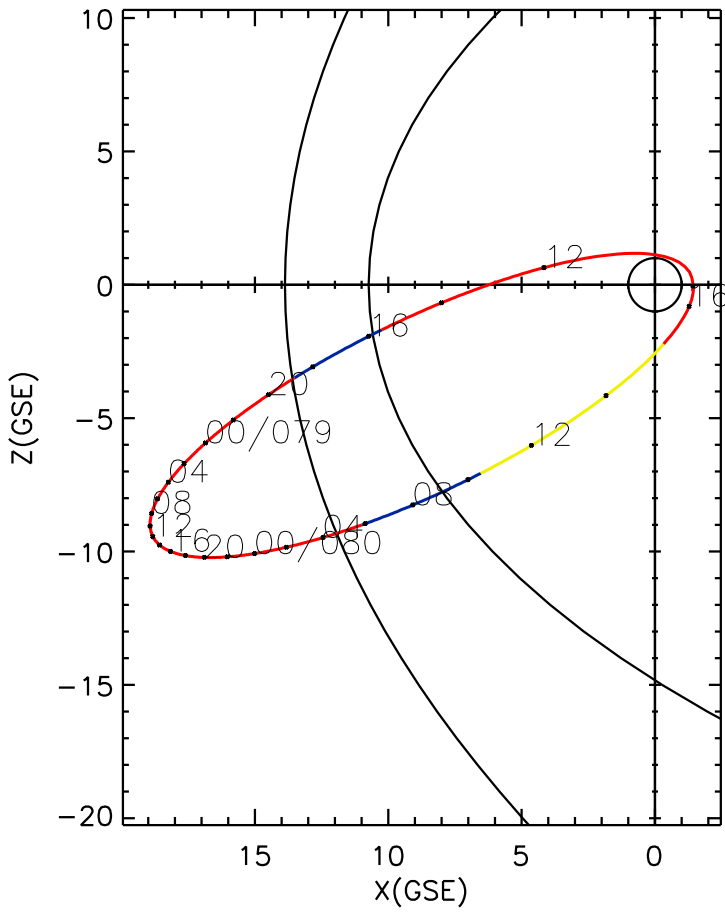
CLUSTER 2 orbit 2010 078 (03/19) 09:56 UT to 2010 080 (03/21) 16:16 UT
