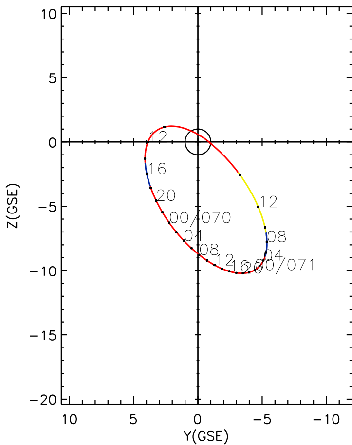
CLUSTER 2 orbit 2010 069 (03/10) 08:46 UT to 2010 071 (03/12) 15:06 UT
